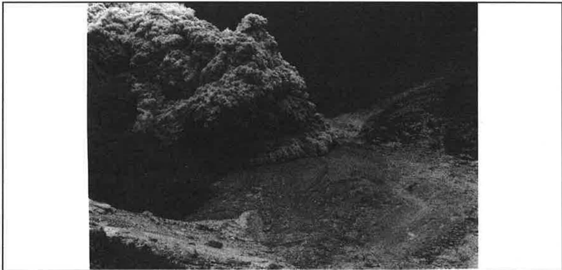
Front nuée ardente du 19.03.92 (photo K.Ohta)
