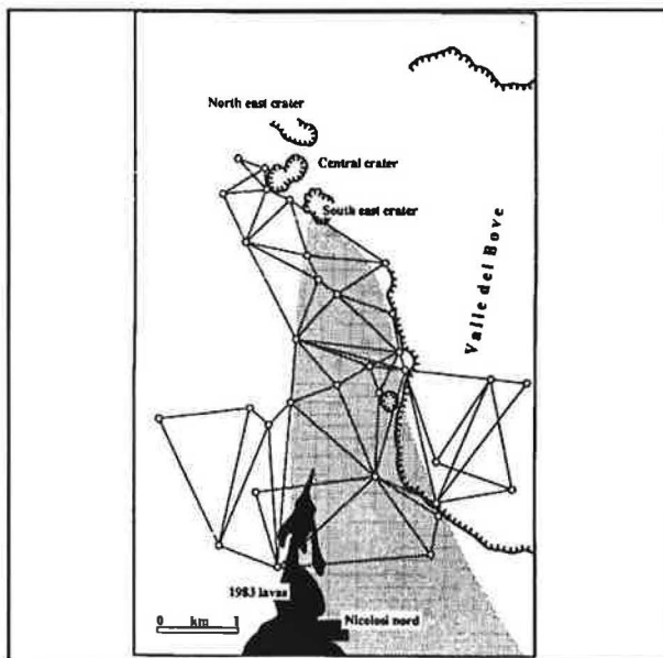
Réseau géodésique, la zone ombrée indique des zones d'intrusions de dykes entre 1981-93 McGuire et al. 1993.
